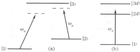
图 1 \Lambda 型三能级原子的能级位形图 (a) 及缀饰态示意图 (b)
