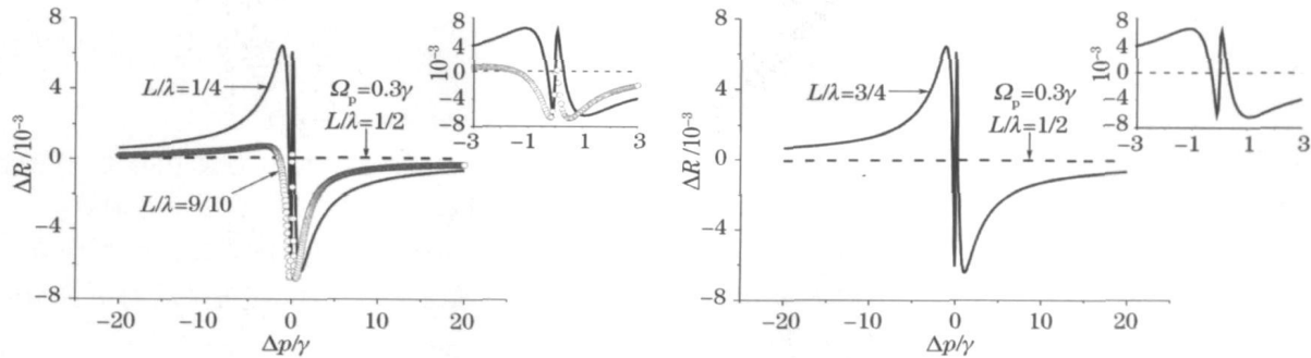
图 3 强抽运光作用下对应不同 L/\lambda 的 TDNSR 线型 Fig.3 TDNSR lines with different L/\lambda for a strong pump field
