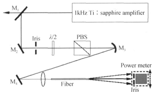
图 1 实验装置 Fig.1 Experimental setup
