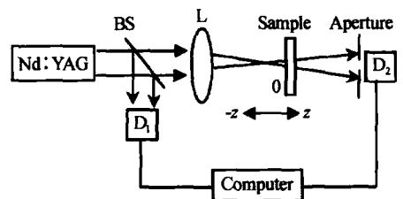
图 1 Z-扫描实验装置 Fig. 1 Setup of the Z scan experiment
