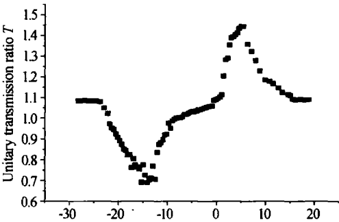
图2 Nd:YVO 4 晶体的Z扫描数据曲线 Fig. 2 Diagram of Nd:YVO 4 crystal Z scan data
