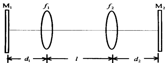
图 2 谐振腔的热透镜等效图
