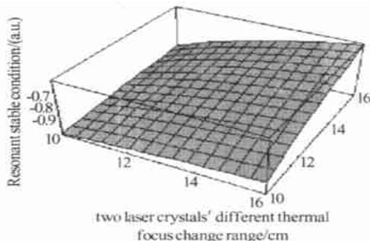
图 4 稳定条件下两个激光晶体热焦距的变化范围
