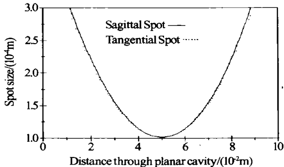
图5 腔内不同距离处光斑的尺寸大小
