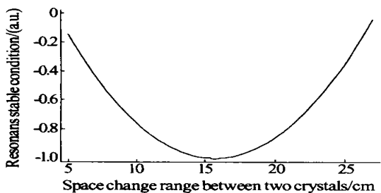
图 3 稳定条件下晶体间距的变化范围
