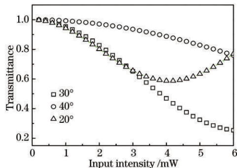
图3 不同偏振夹角下透射率变化模拟曲线
