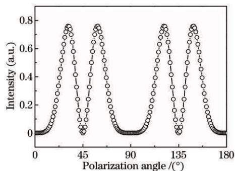
图2 偏振椭圆旋转效应强度随偏振夹角变化的模拟曲线
